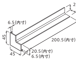
入隅カバー 製品図
