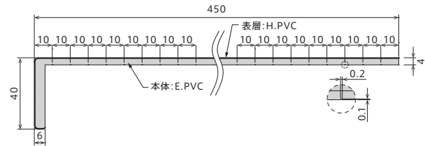
マルチユース窓枠カバー450 製品図
