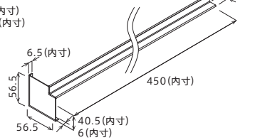
入隅カバー450 製品図
