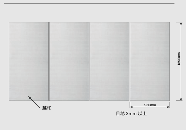
施工補助部材を使用しない場合の例
