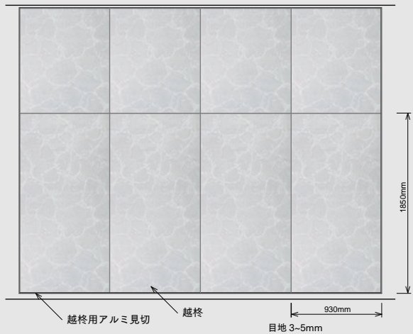
施工補助部材を使用する場合の例
