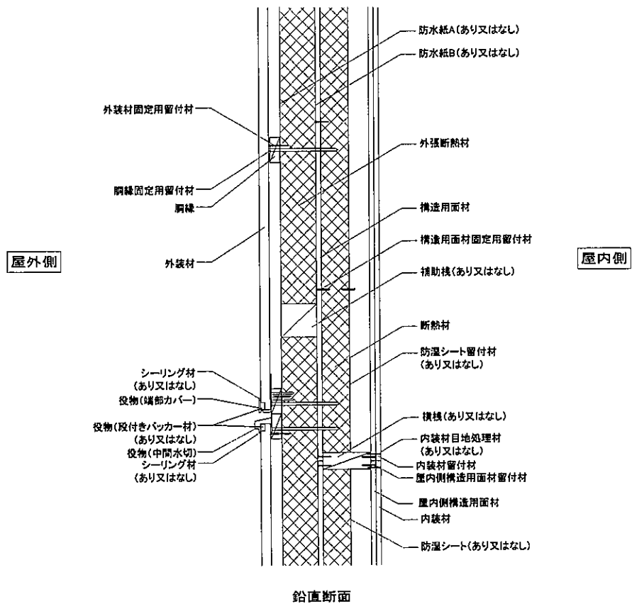
鉛直断面
