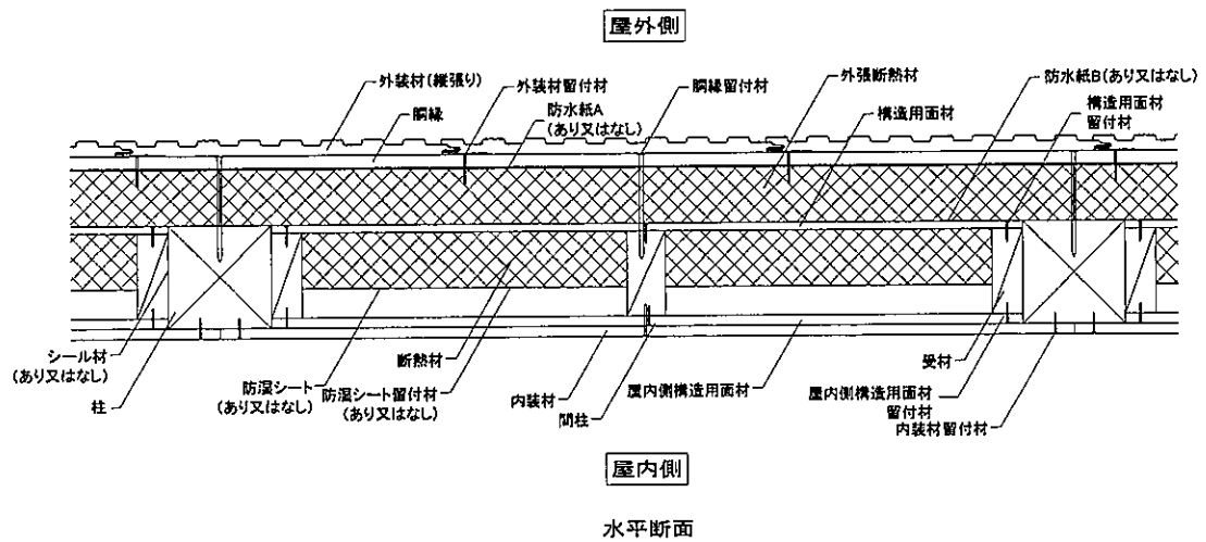
水平断面
