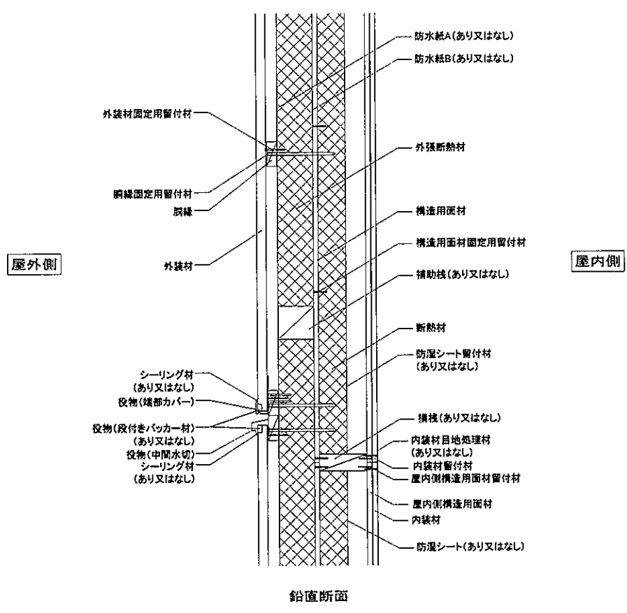
図2 構造説明図 (構造用面材(屋外側大壁、屋内側大壁))
