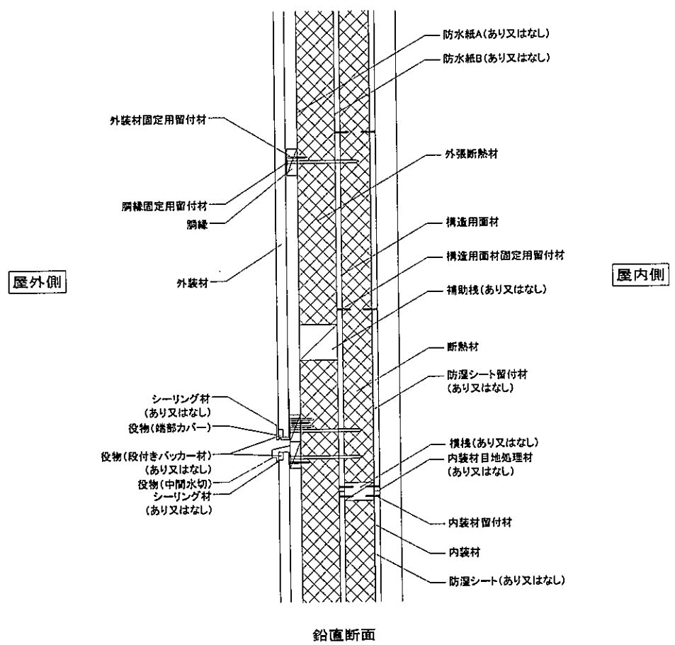
図18 構造説明図 (構造用面材(屋外側真壁(受材仕様)、屋内側真壁(切り欠き仕様)))
