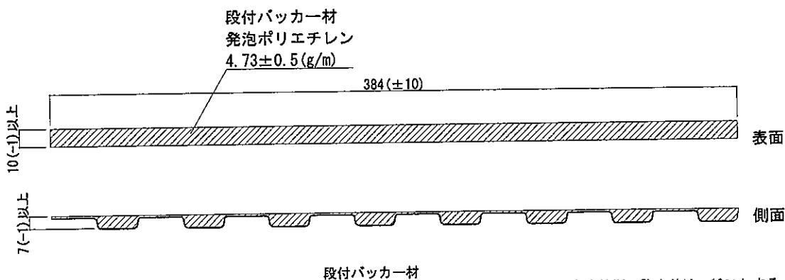
図19 構造説明図
