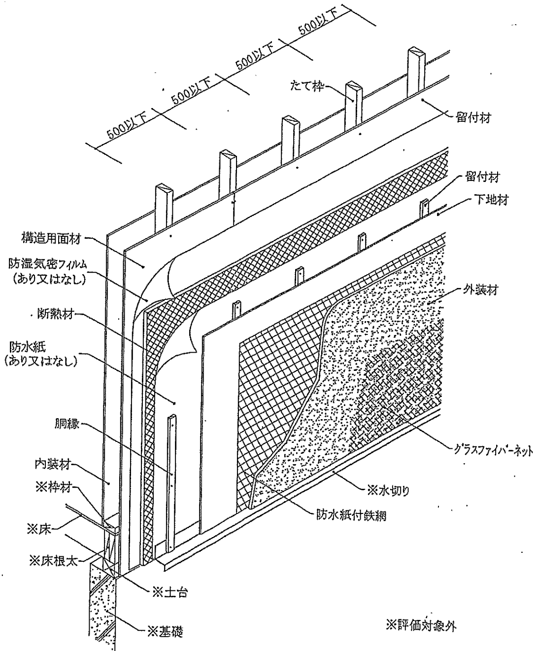
透視図
