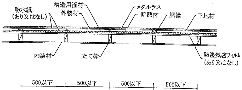
水平断面図
