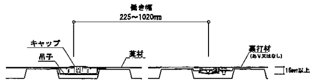
葺材断面 (代表的な仕様)
