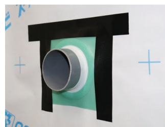
パイプ用 パイプ周りの防水テープは不要!
